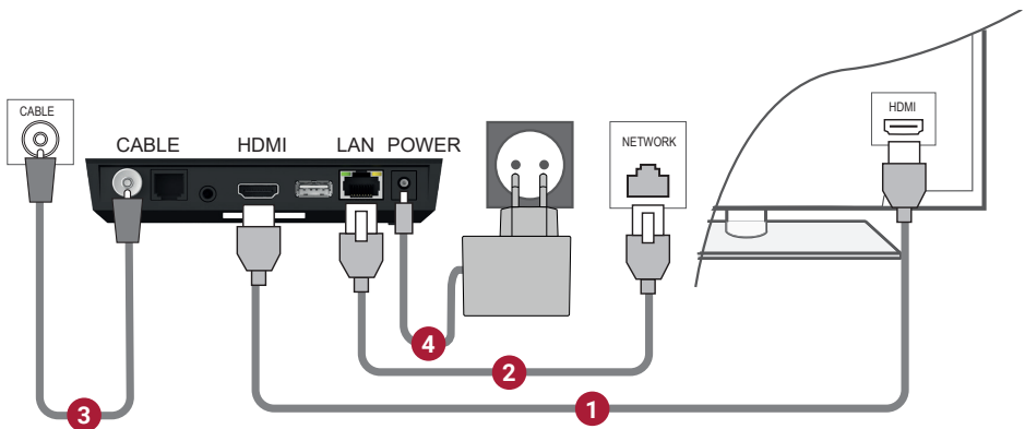
Abbildung 3: Kabelverbindungen
